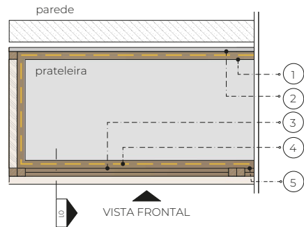
PLANTA BAIXA
