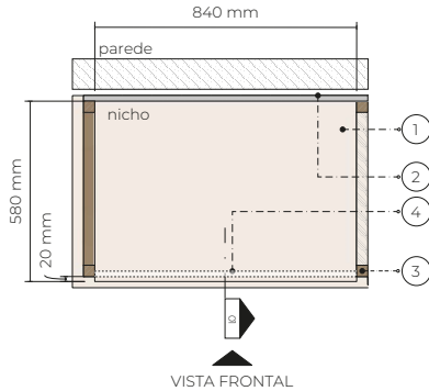
PLANTA BAIXA
